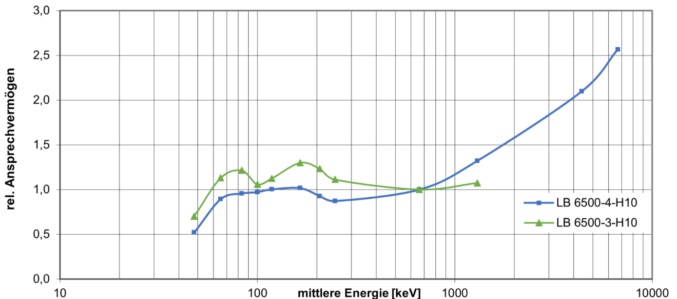
Energieabhängigkeit LB 6500-4-H10 und LB 6500-3-H10
